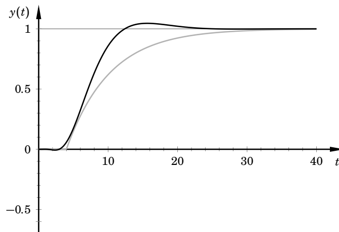
Figur 6.7 Stegvar för processen i problem 6.10
