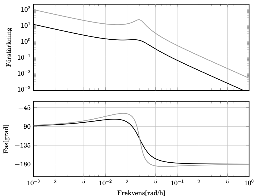
Figur S8.1 Bodediagram för den PD-komenserade öppna loopen i uppgift 8.1. De svarta kurvorna svarar mot hastigheten v = 3 knop (nominella fallet) medan de gråa kurvorna visar fallet v = 7 knop. Notera att det senare fallet ger ett instabilt slutet system.
