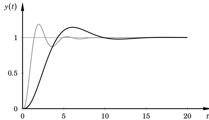
Figur S6.11 Stegsvär för slutet okompenserat (heldragen kurva) och kompenenserat system (streckad kurva) i problem 6.14.
