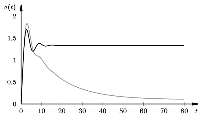
Figur S6.18 Rampfel för det slutna okompenserade (svart linje) och kompenserade (grå linje) systemet i problem 6.16.
