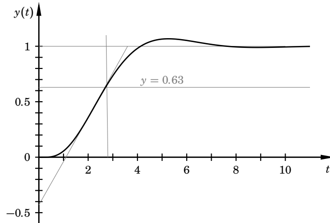
Figur S6.3 Stegsvär för systemet i uppgift 6.8 med några intressanta linjer inlagda
