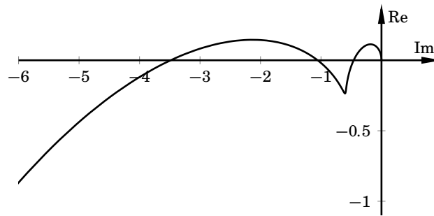
Figur 4.2 Nyquistkurva för systemet i uppgift 4.14.
