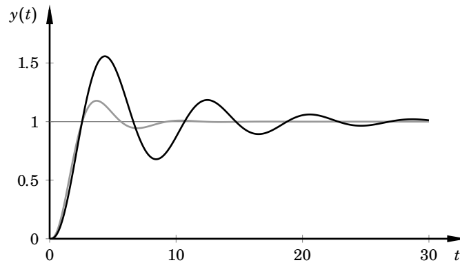
Figur S6.14 Stegsvär hos det slutna okompenserade (svart linje) och kompenserade systemet (grå linje) i problem 6.15.
