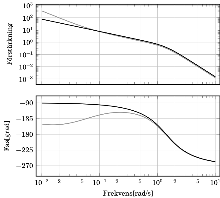
Figur S6.16 Bodediagram för det öppna okompenserade systemet (svart linje) och för det öppna kompenserade systemet (grå linje) i problem 6.16.
