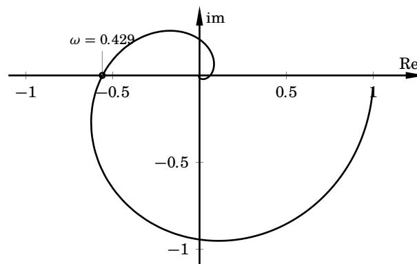
Figur 6.8 Nyquist-diagram för processen i problem 6.10
