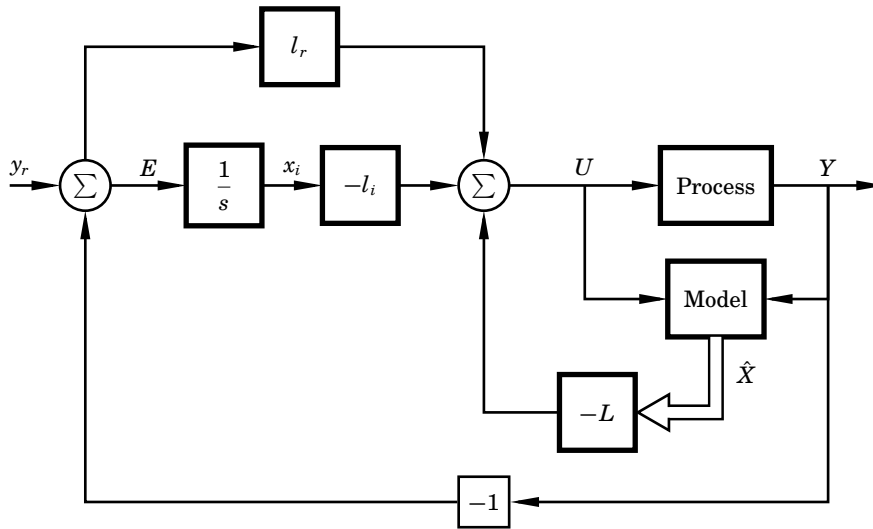
Figur 8.8 Blockschemata för Kalmanfiltrering med tillståndsåterkoppling i uppgift 8.2.
