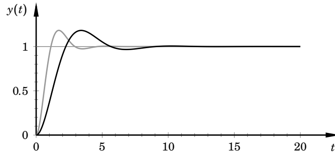
Figur S6.9 Stegsvär hos det slutna okompenserade (svart linje) och det kompenserade (grå linje) systemet i problem 6.13.
