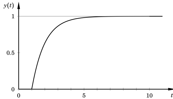
Figur S6.4 Stegsvär för G(s) = e^{-s}/(s+1) .
