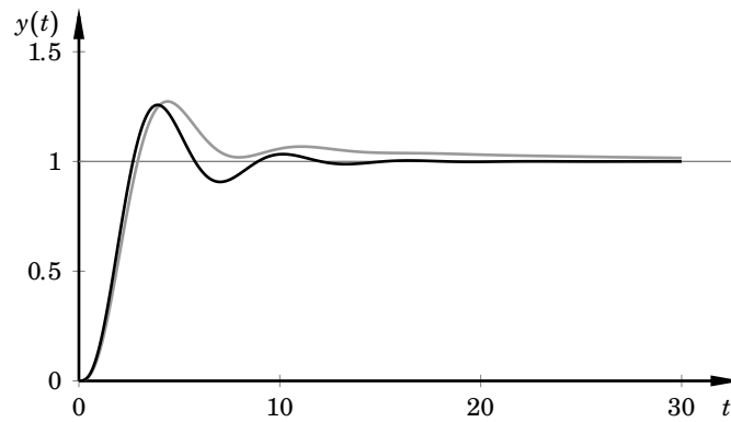
Figur S6.17 Stegsvär för det slutna okompenserade (svart linje) respektive kompenserade systemet (grå linje) i problem 6.16.
