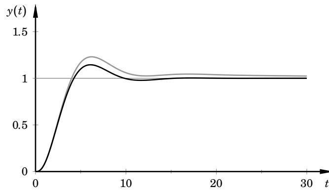
Figur S6.6 Stegsvär hos det slutna okompenserade systemet (svart linje) och det kompen­serade (grå linje) systemet i problem 6.12.
