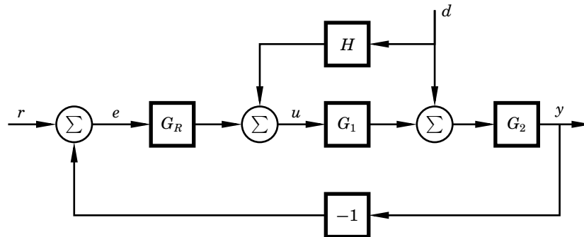
Figur 7.1 Blockschema för temperaturreglering av hus.
