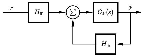
Figur 7.4 Ekvivalent blockschema för uppgift 7.3.
